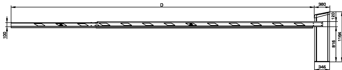
Eksempel på ACCESS bomsystem med 10 m bomlængde:
